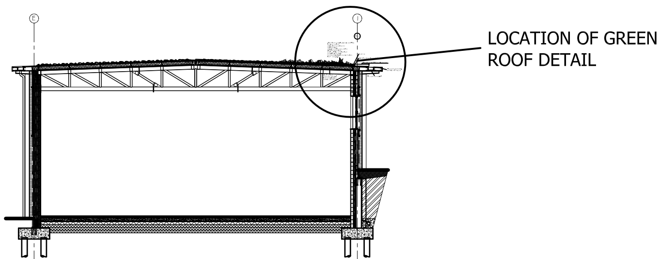
SECTION A-A 1:200
