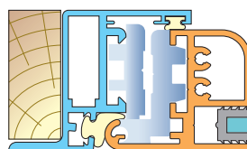
JAMB DETAIL (HINGE)
