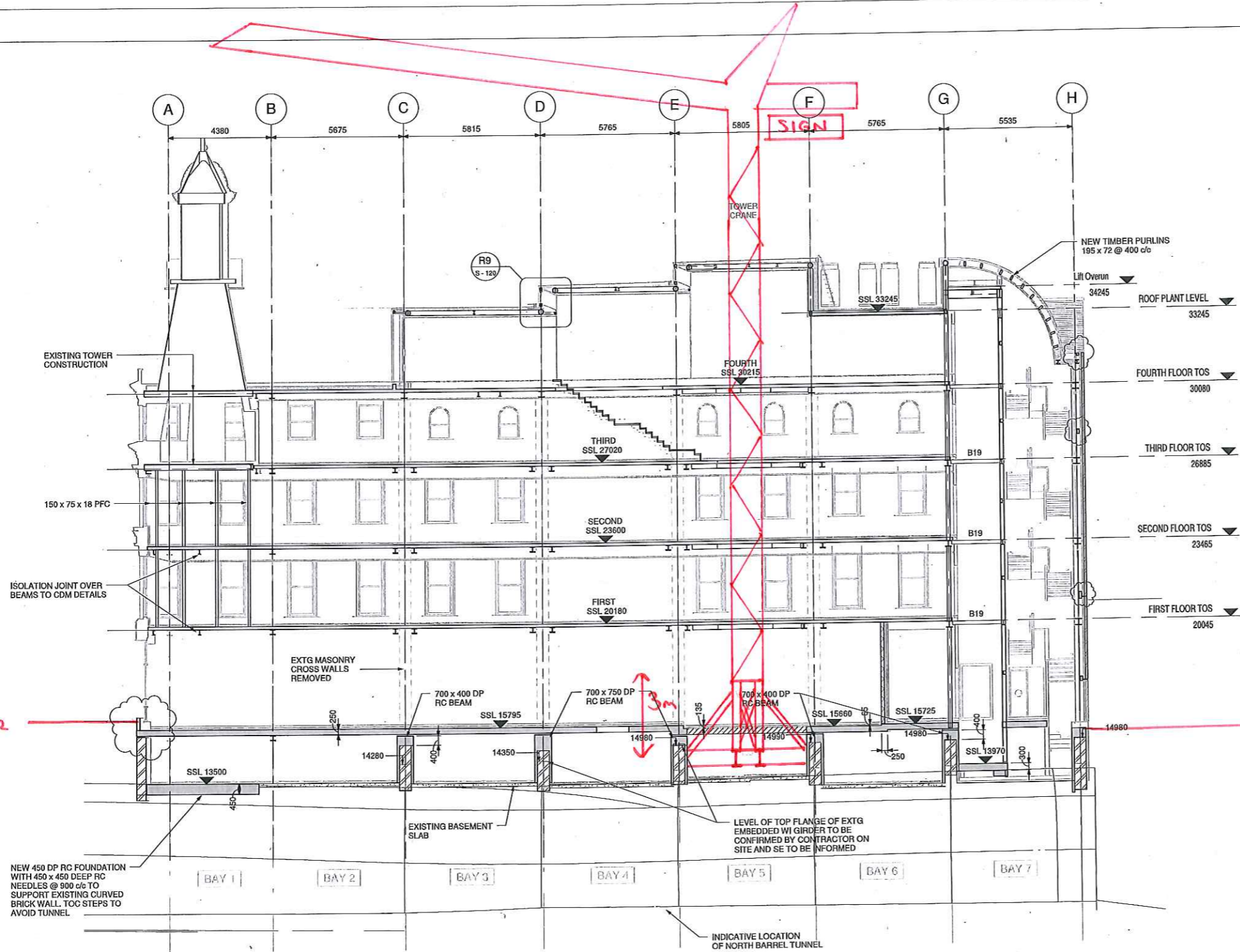
1 Section 1-1 1:100
