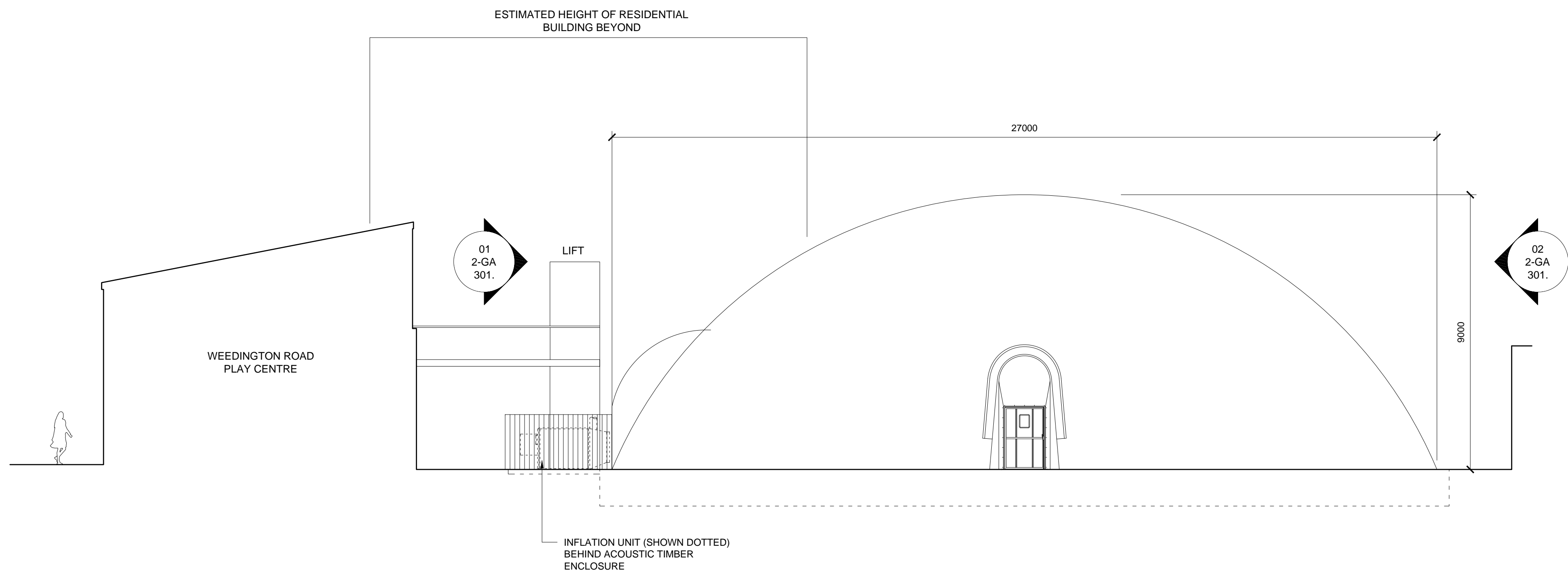
02 ELEVATION @ A1 1:100
