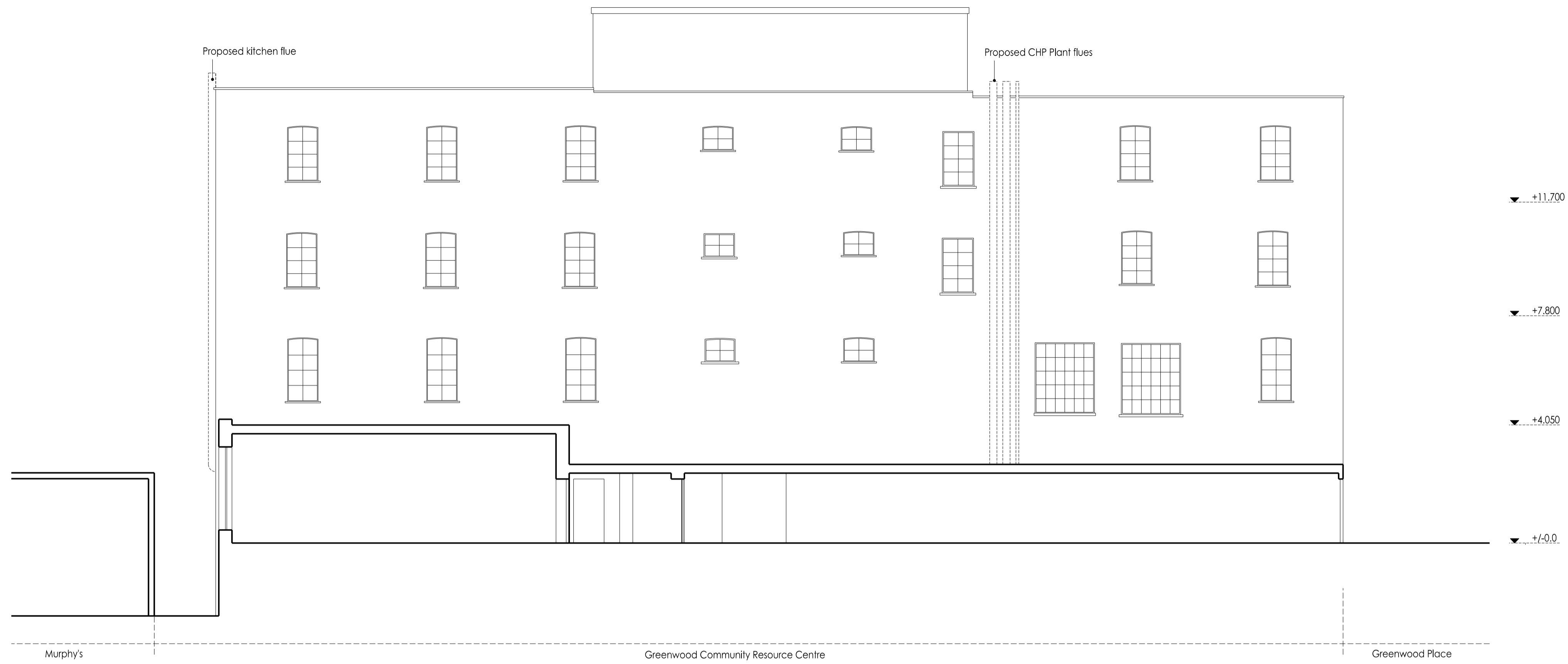
SECTION A-A
