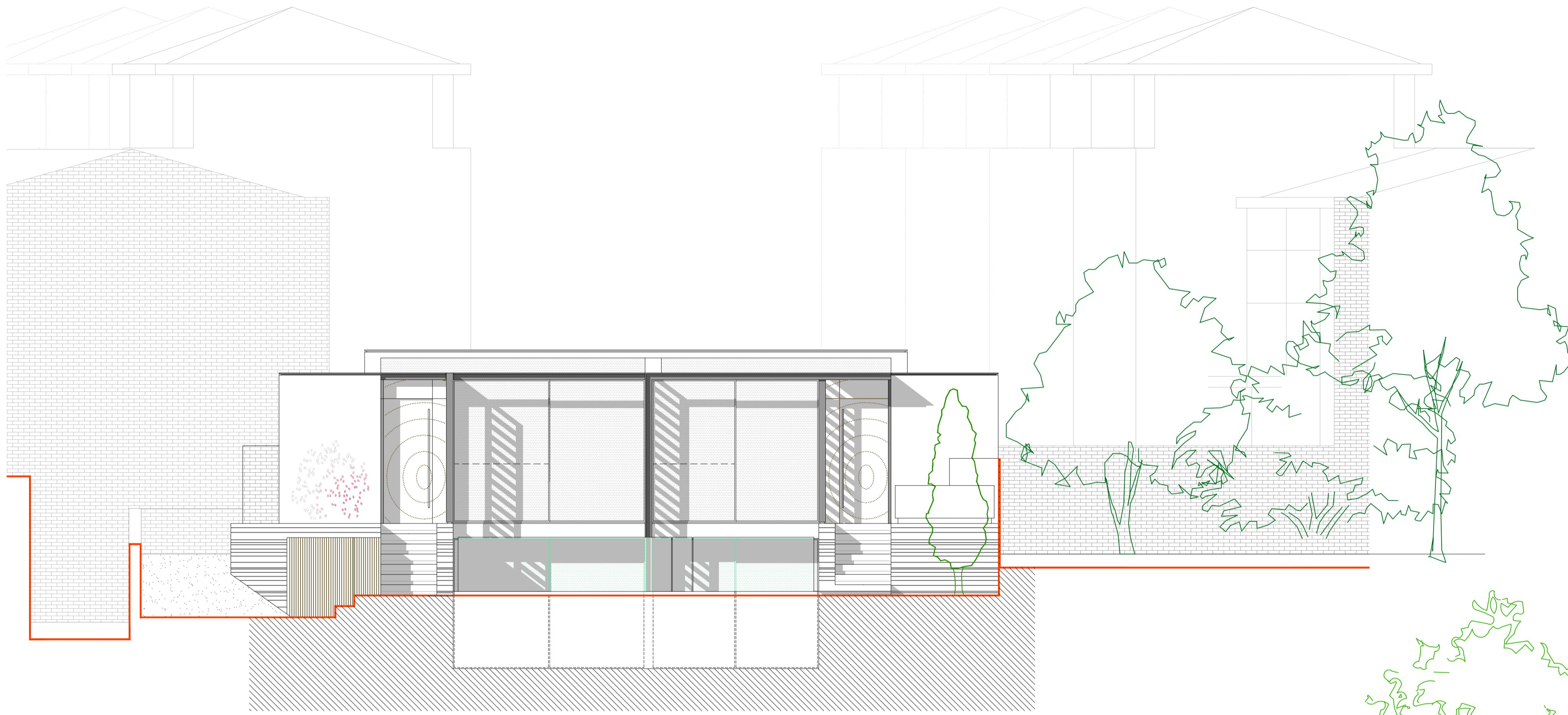
SE ELEVATION
