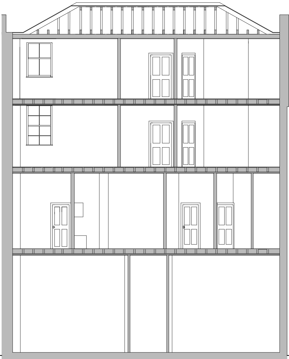
SECTION A-A
