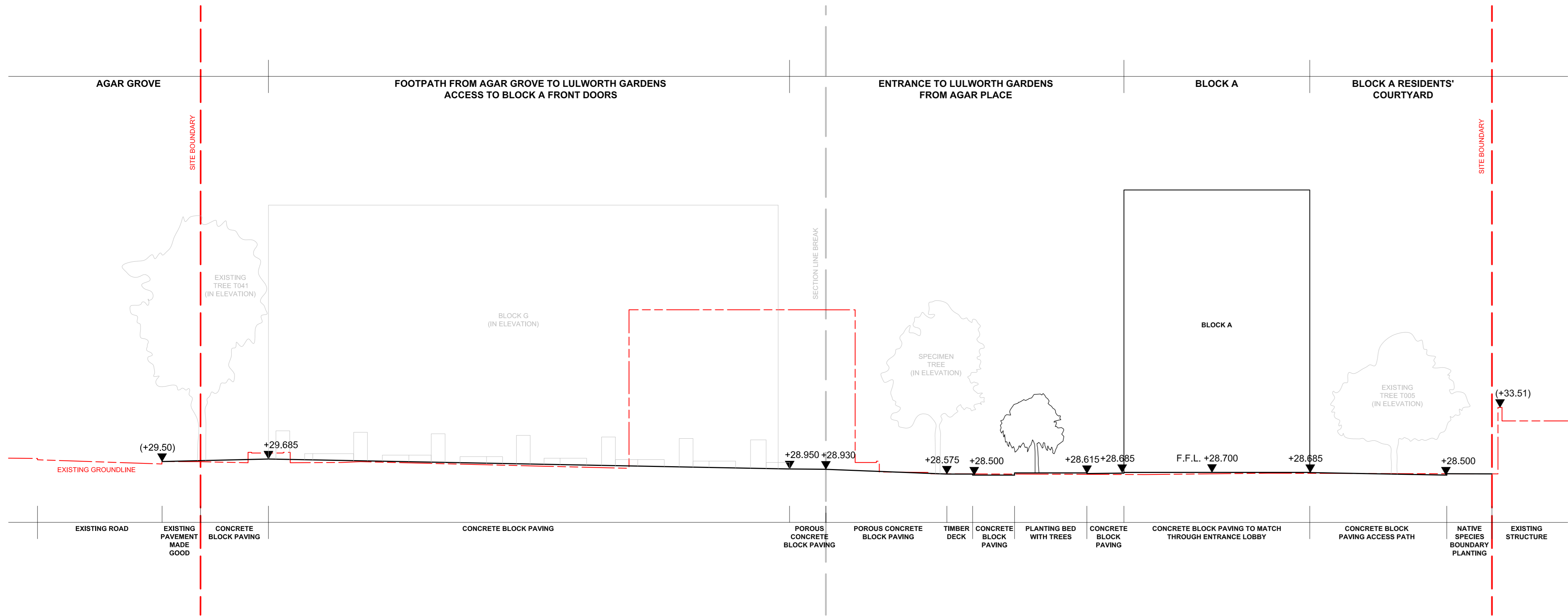
A-A Section Scale 1:200
