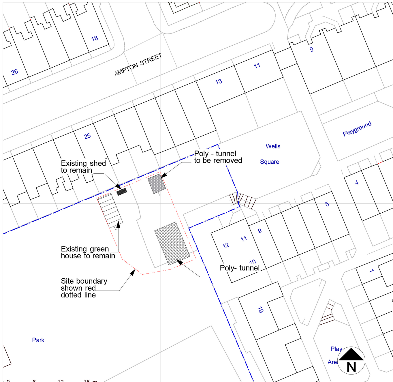
Site Plan 1:500
