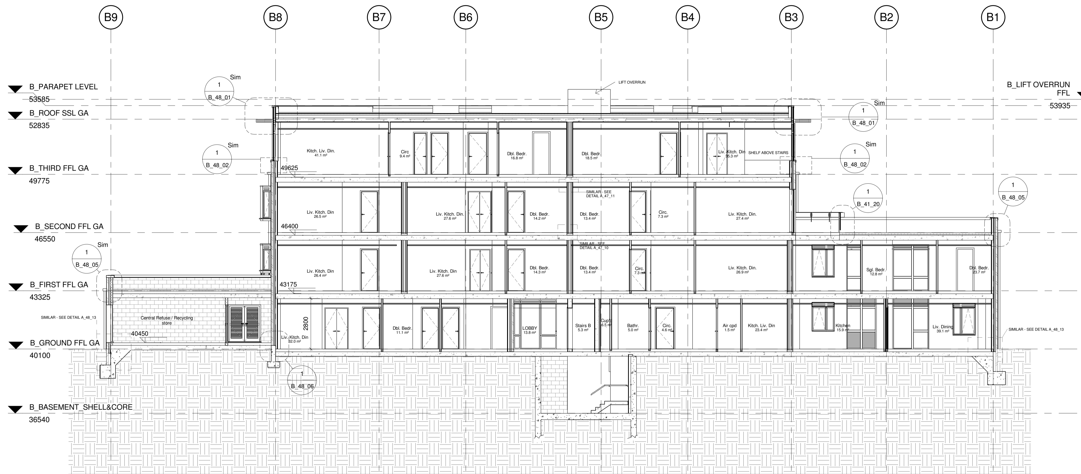
B_SECTION A-A 1 : 100
