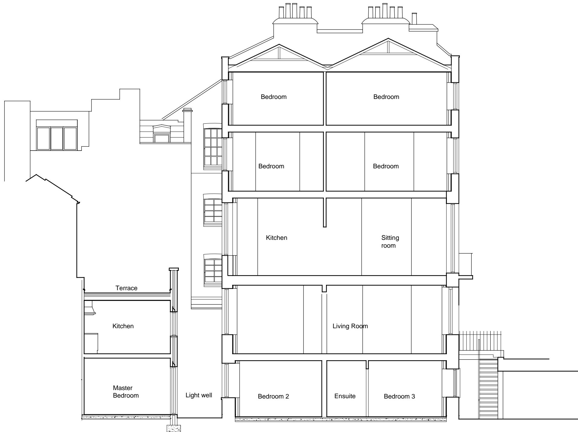
Section D-D
