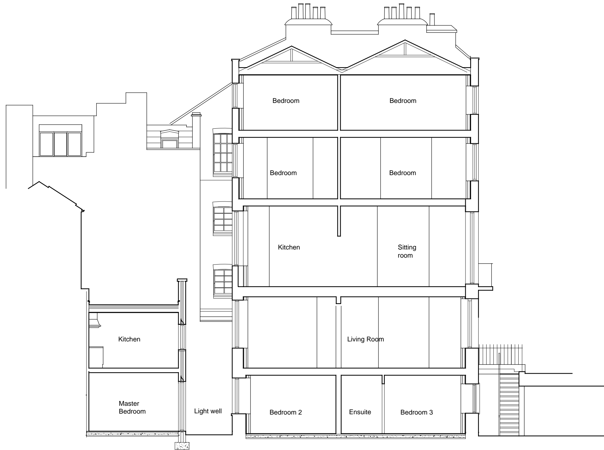
Section D-D
