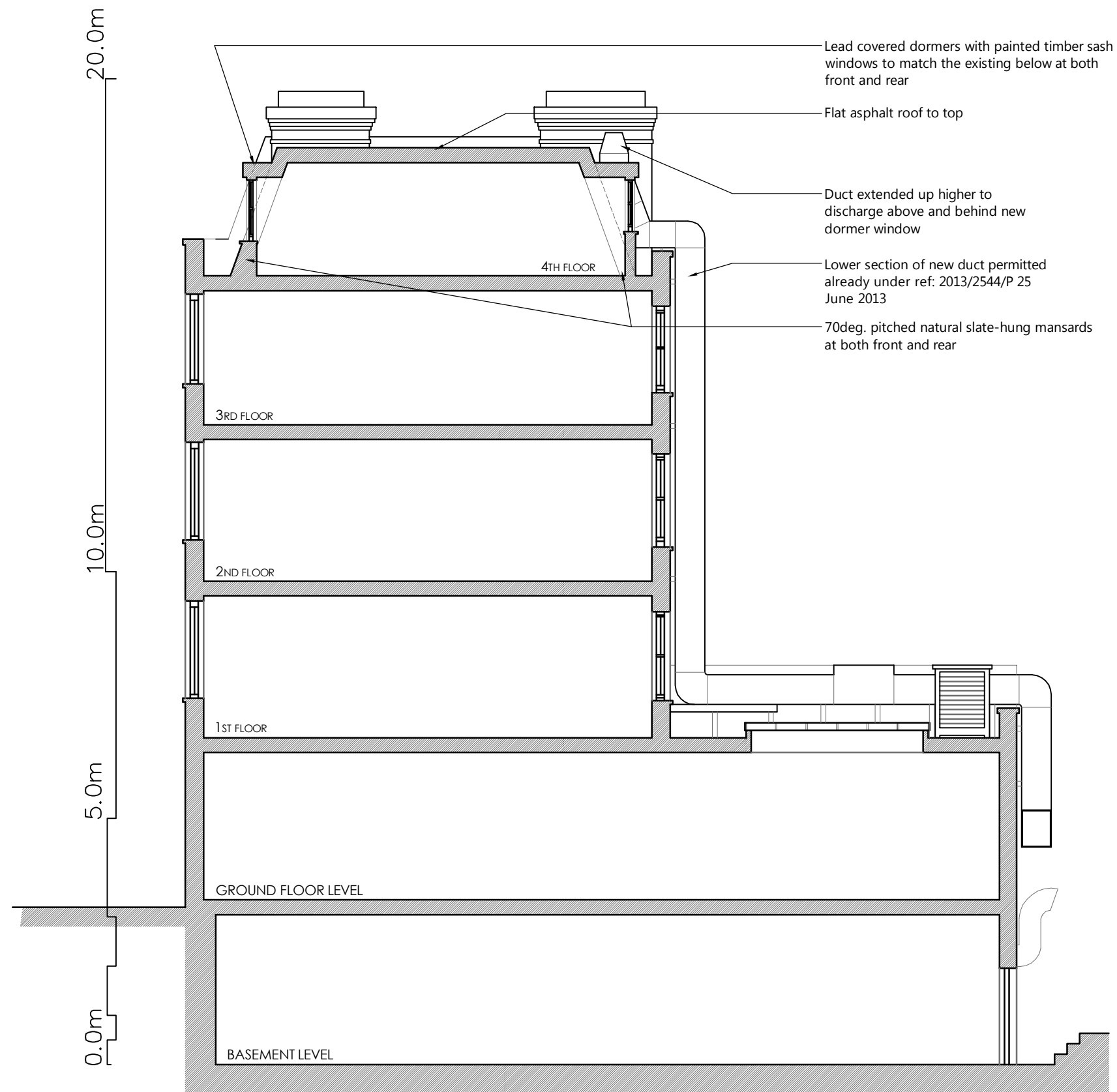
SECTION A-A
