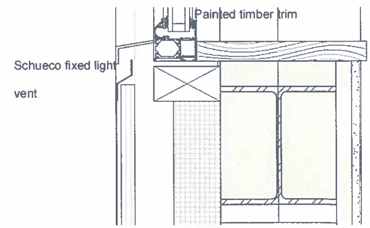
4 fixed light cill Scale: 1:5
