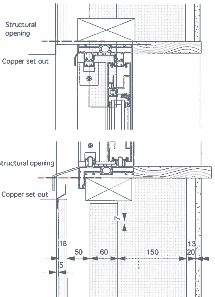
4 Window Head Scale: 1:5
