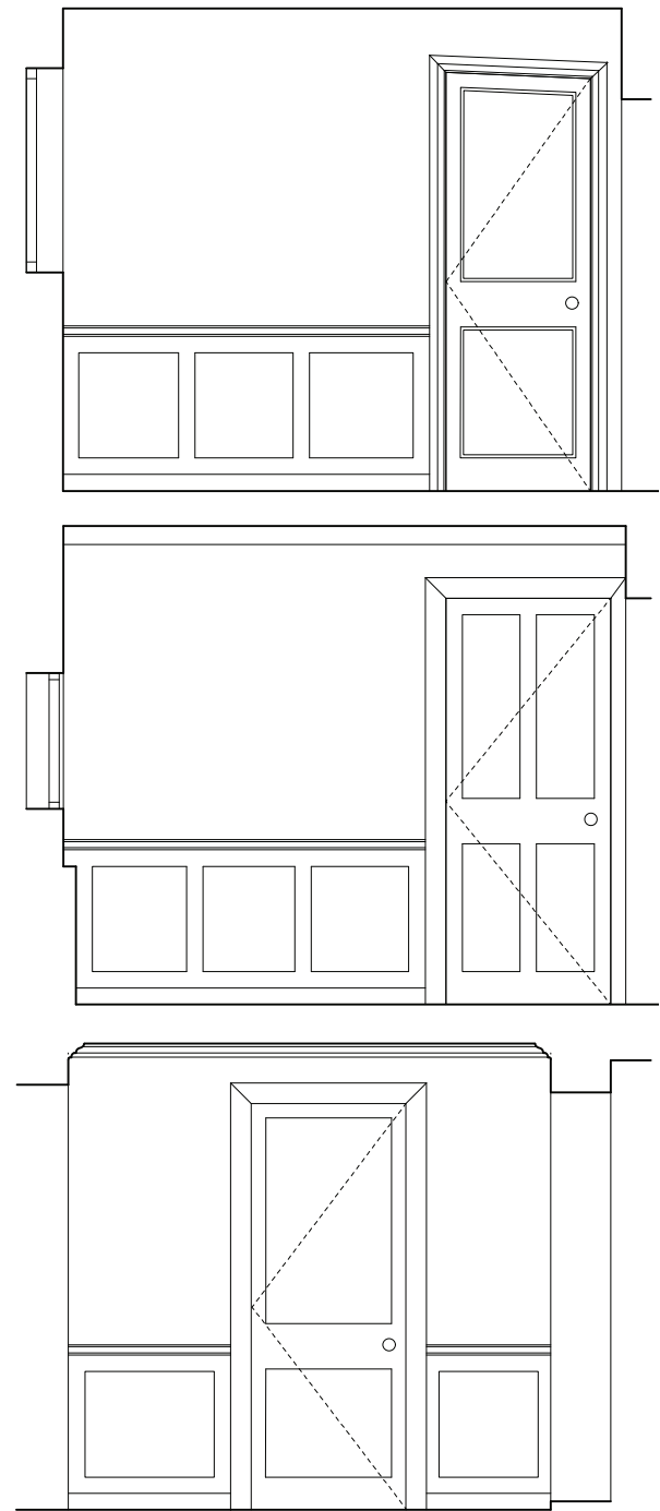
07 Elevation D 1:20@A3
