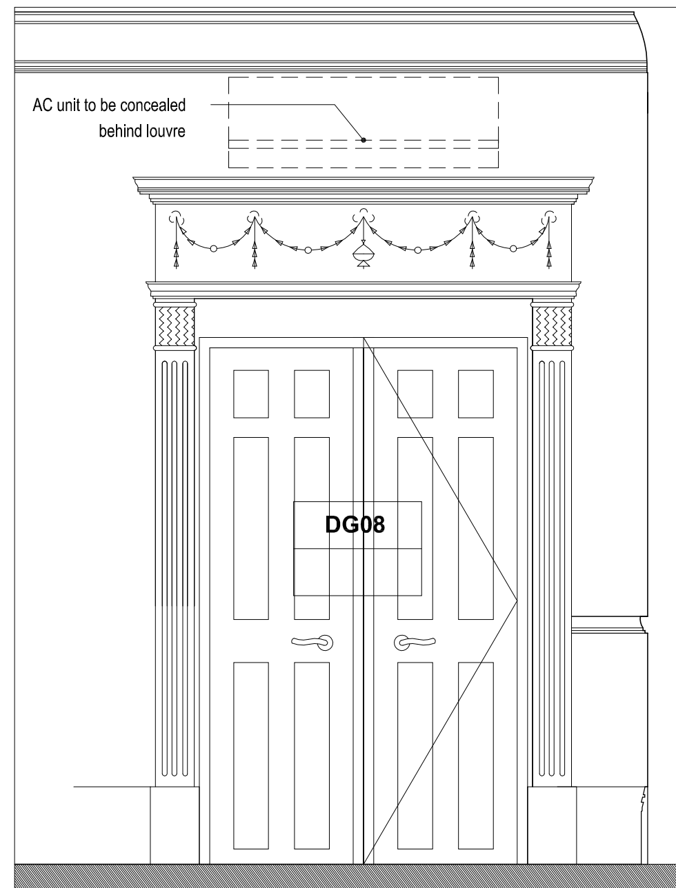
Elevation
