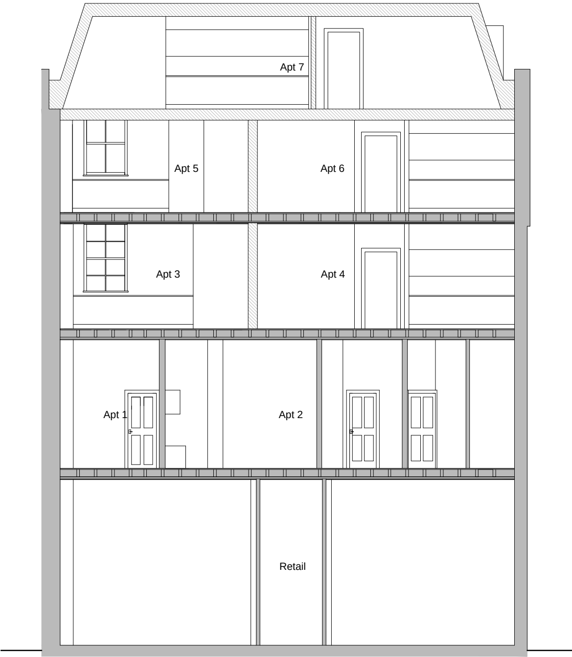
SECTION A-A
