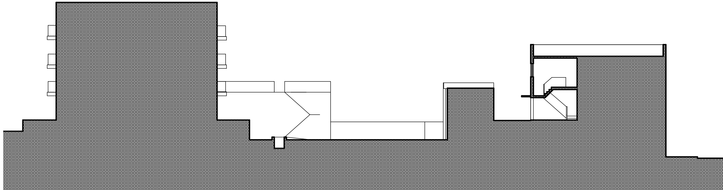
1 existing section AA Scale: 1:200
