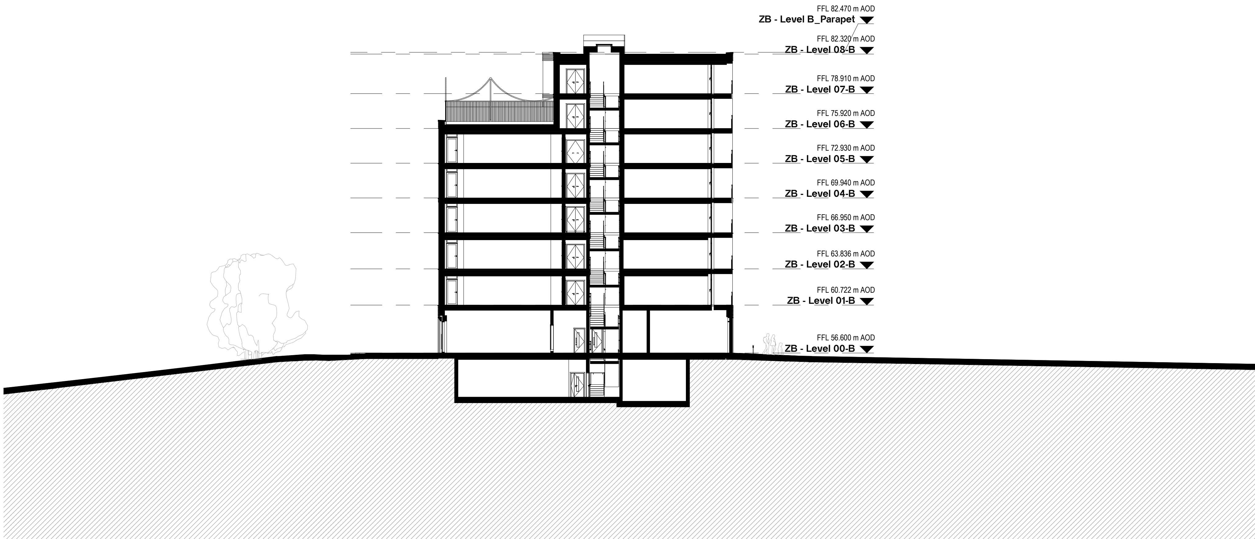
Section E-E 1 : 200
