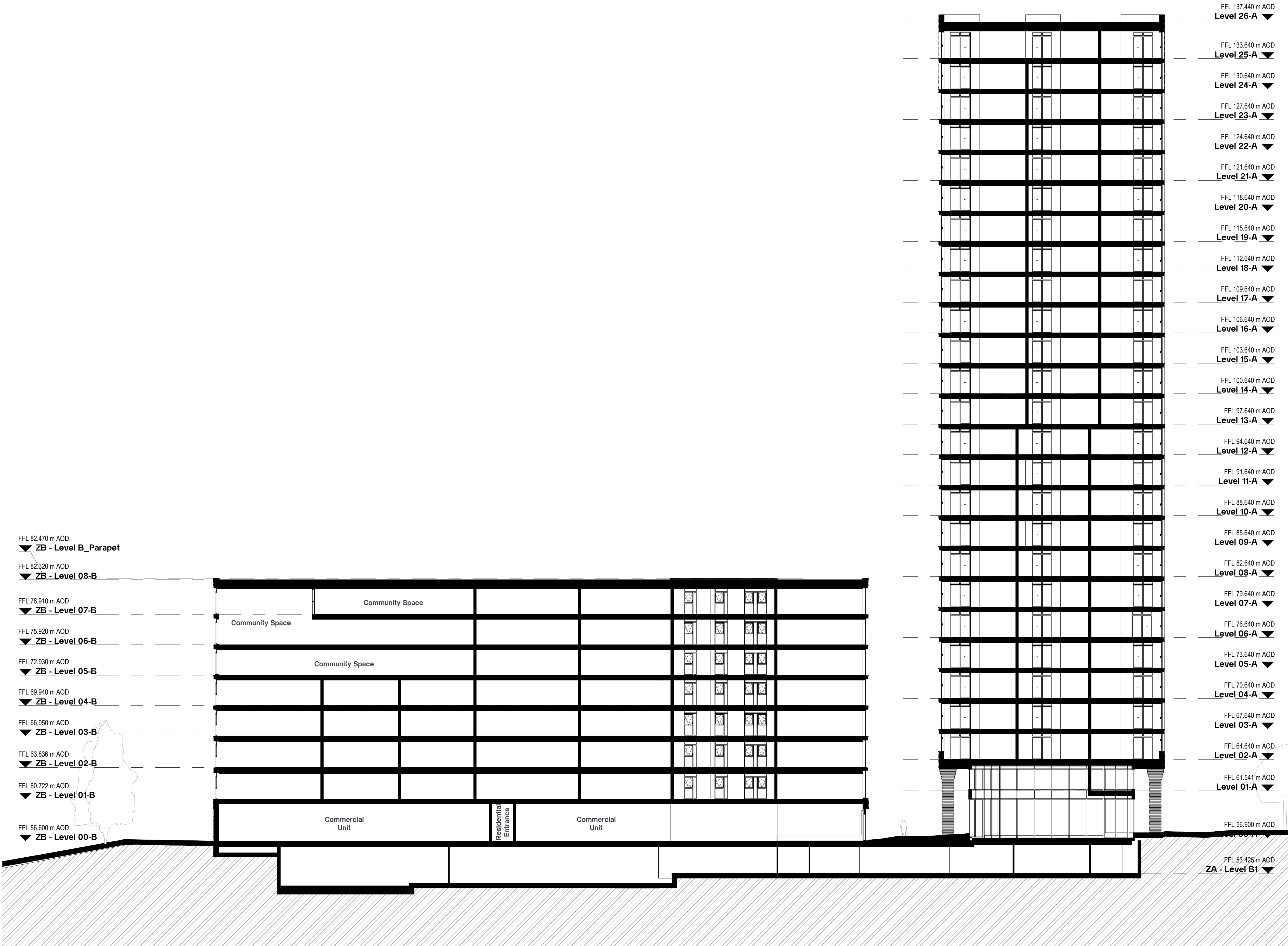
Section C-C 1 : 200
