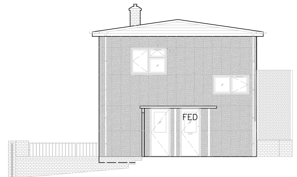
Existing Flank Elevation
