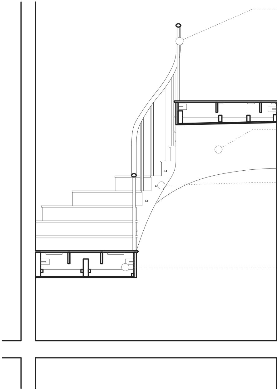
Section A-A
