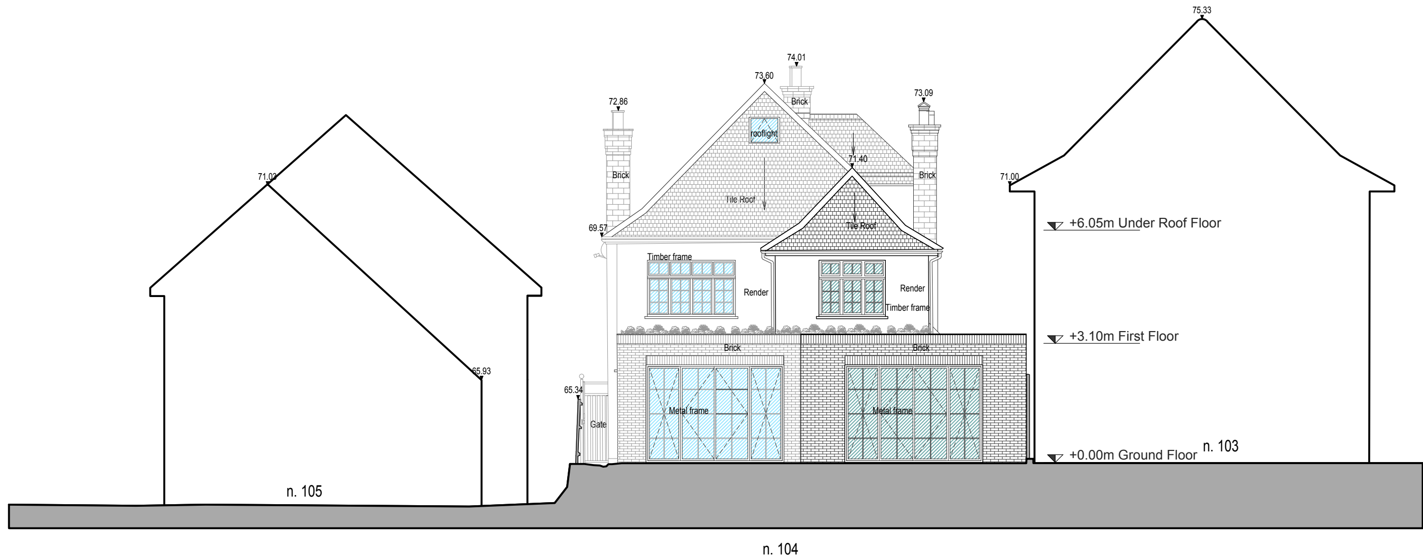
ELEVATION 3
