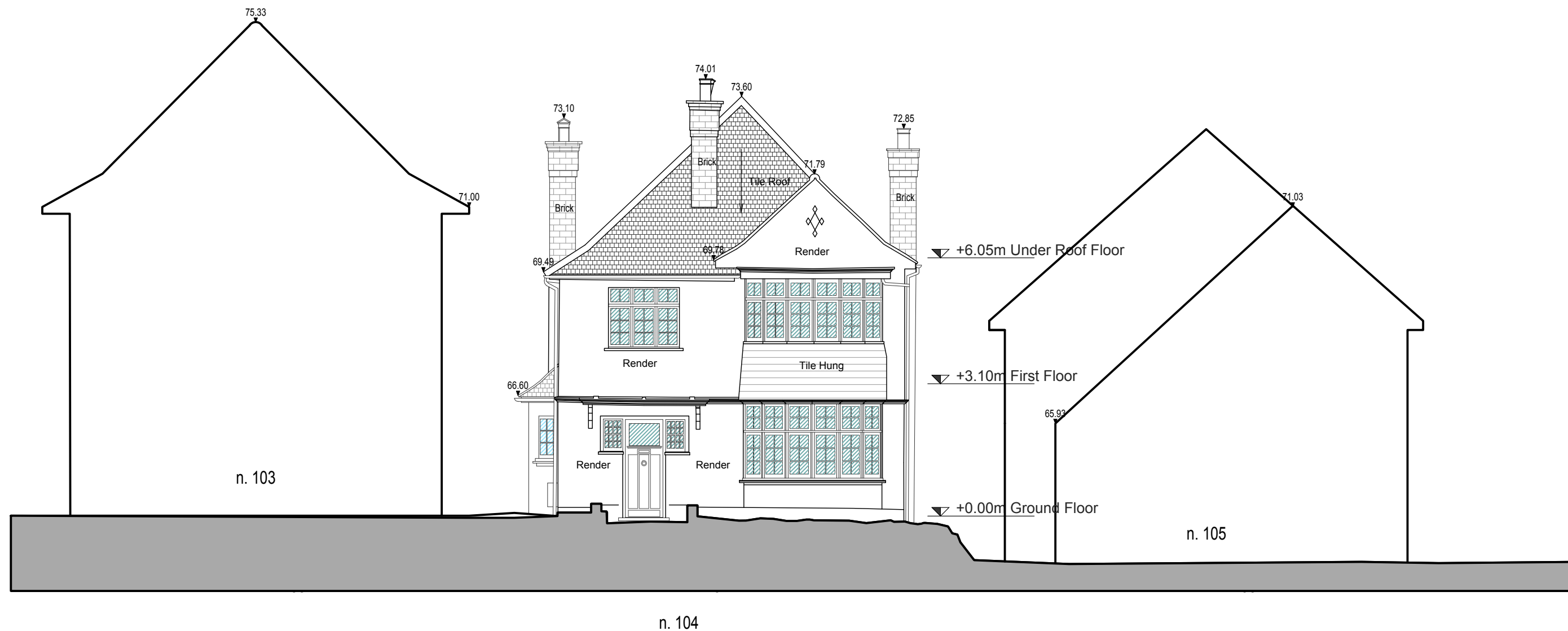
ELEVATION 1
