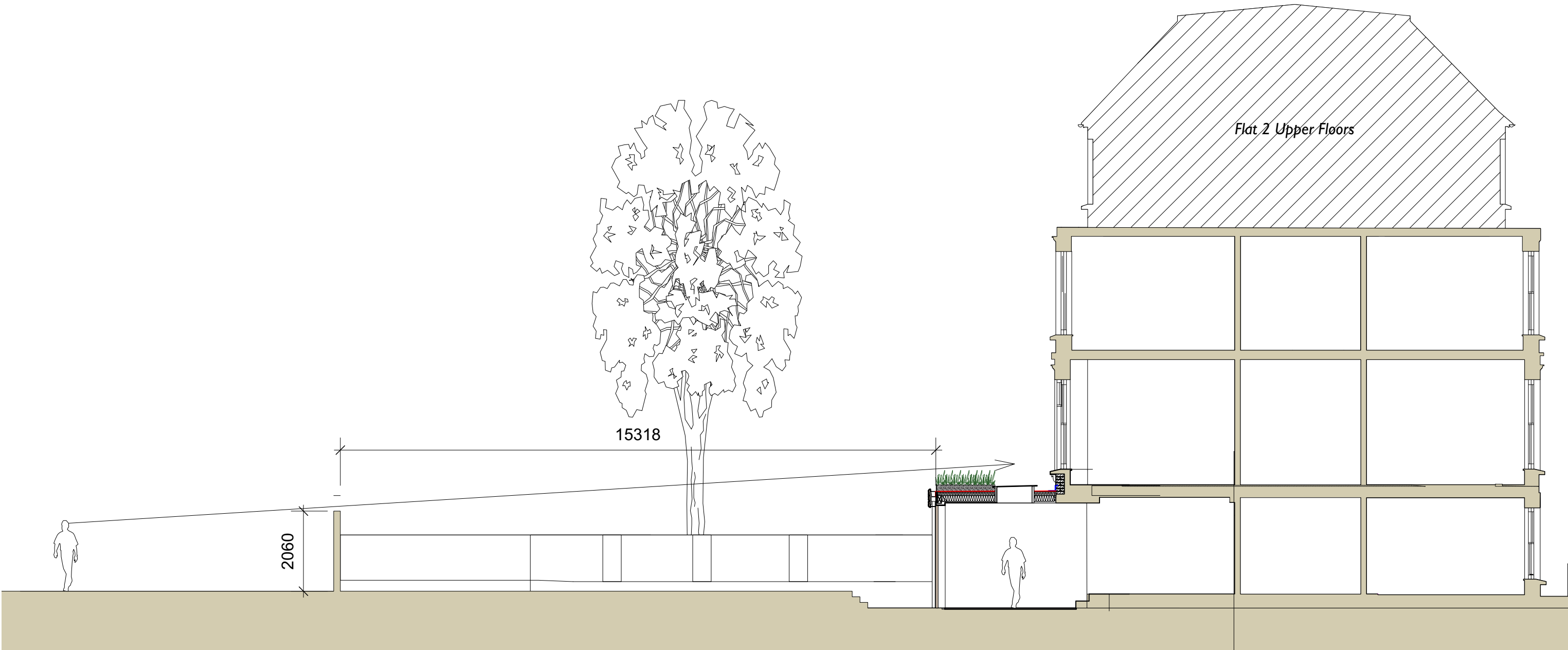
2 Section AA Scale: 1:100
