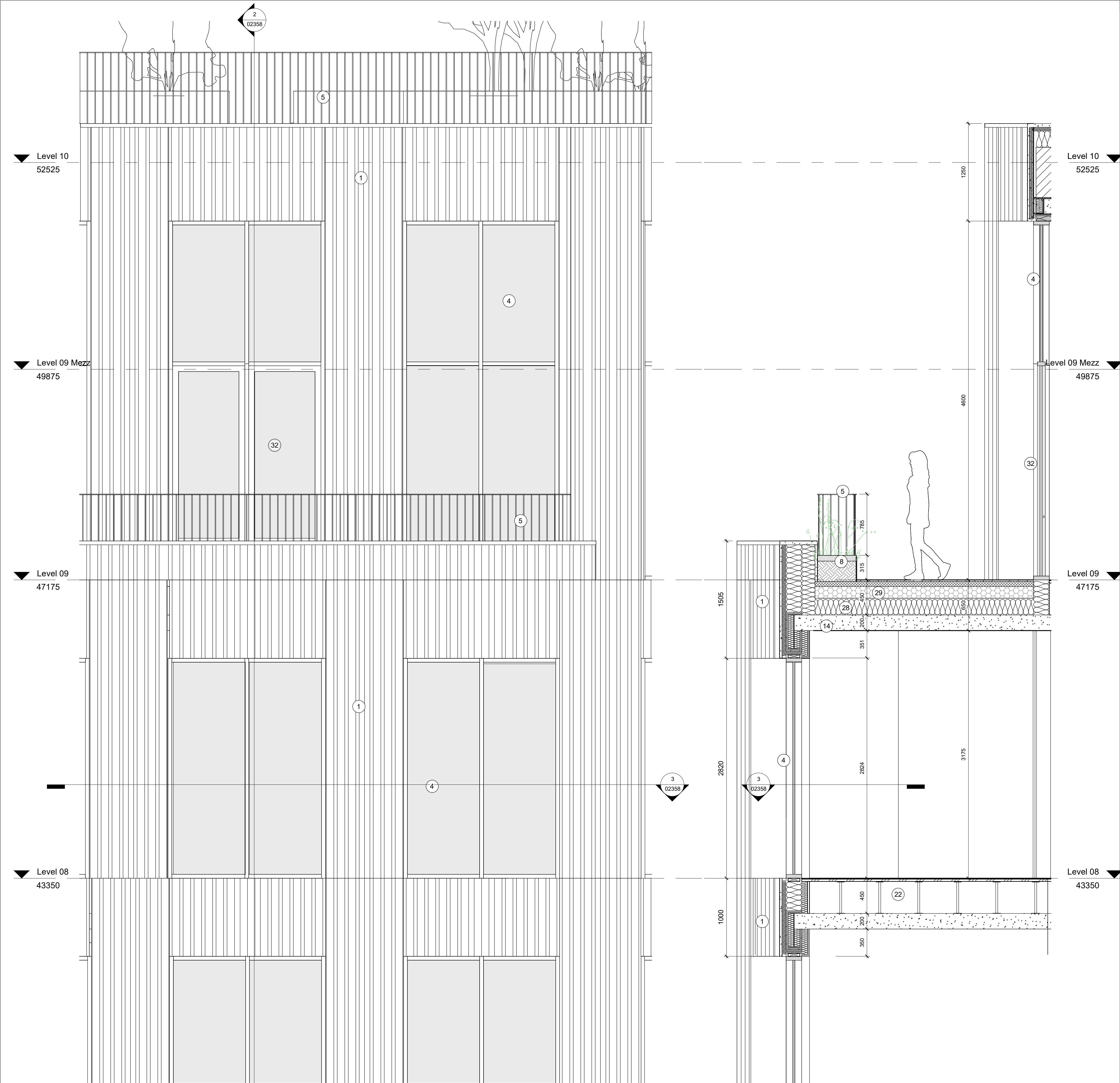
1 Elevation SH Top 1 : 25
