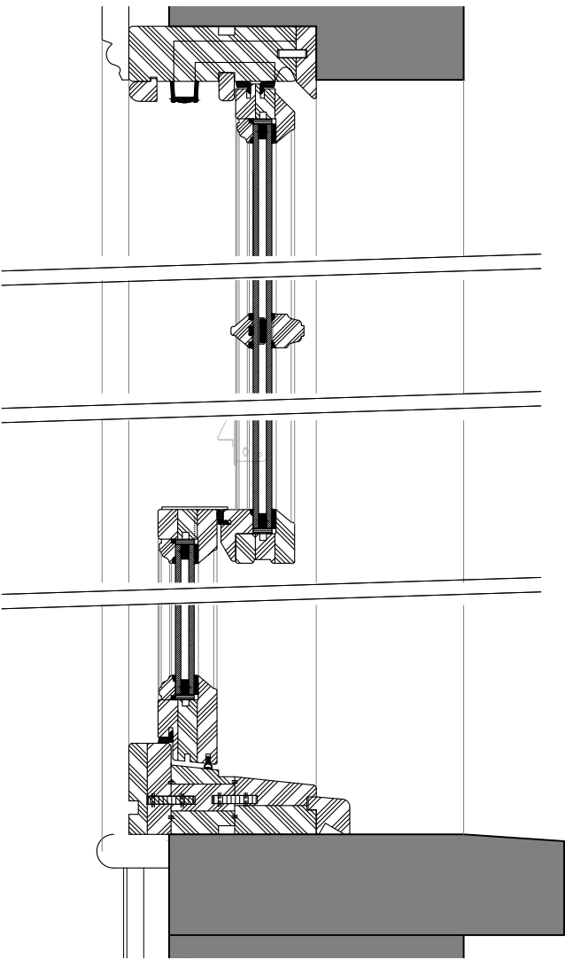
SECTION A-A – 1:5
