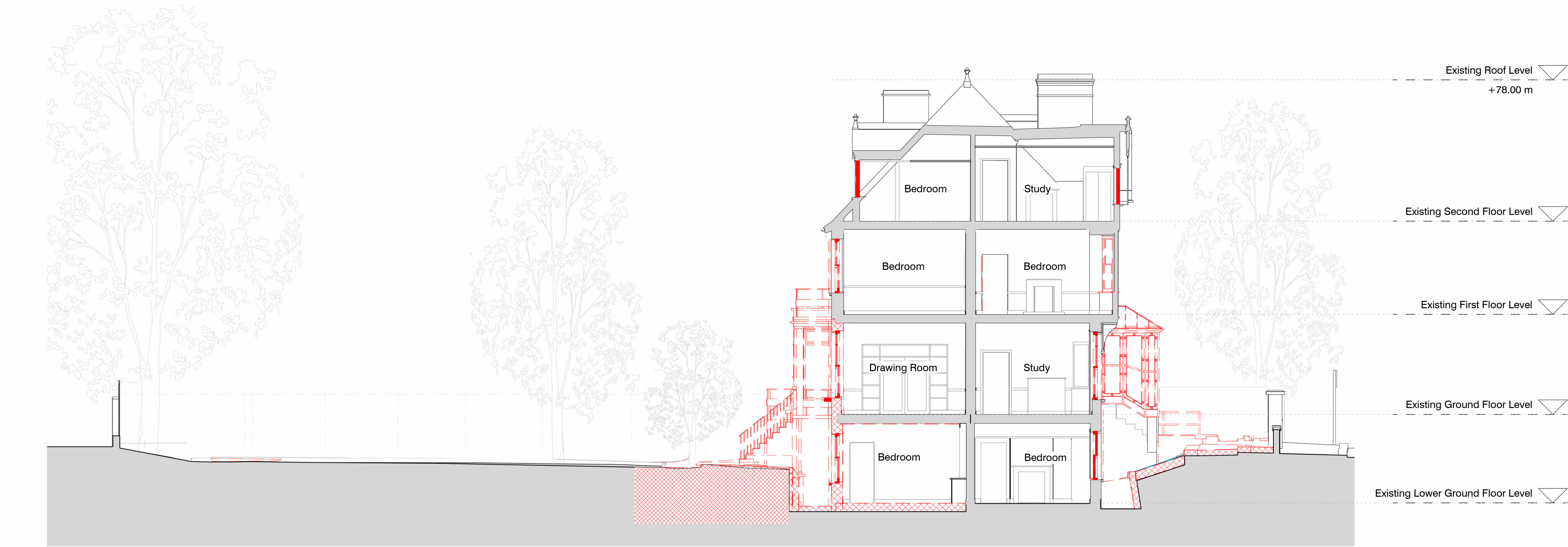
1 Demolition Section AA P_2200 1 : 100
