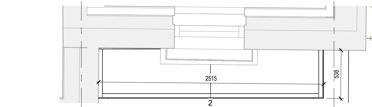
1 External Canopy Plan 1 : 25
