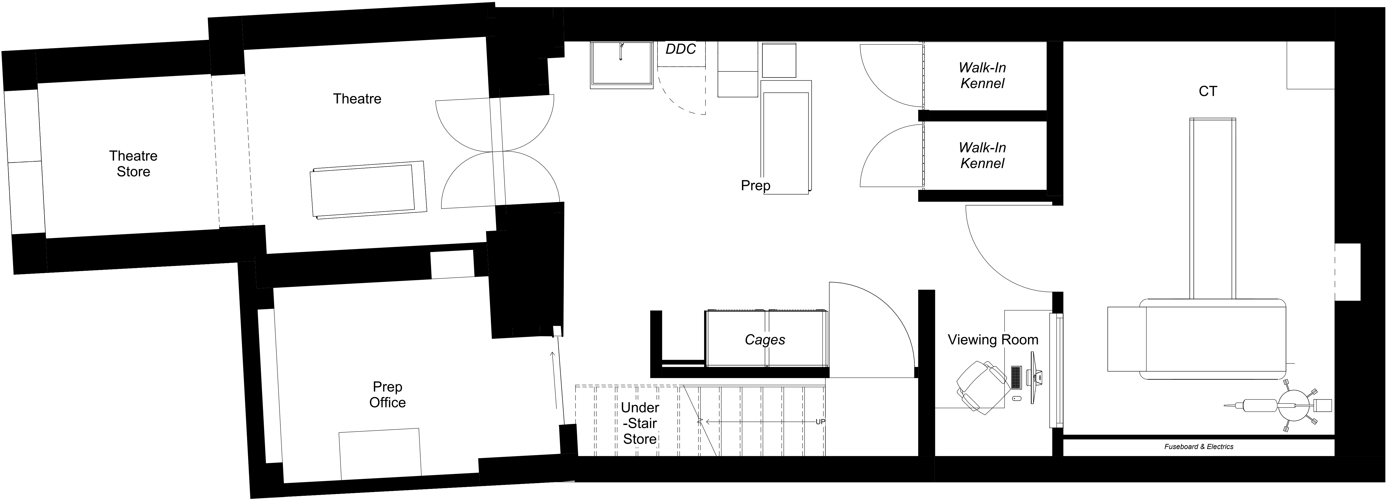
0.0 Basement - Existing 1 : 25
