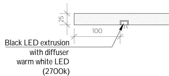
Detail O2 - 1:5
