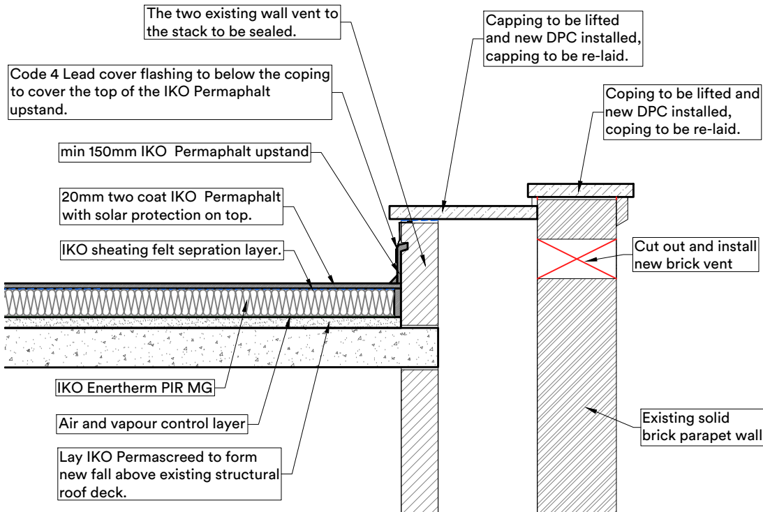
Section S1-S1
