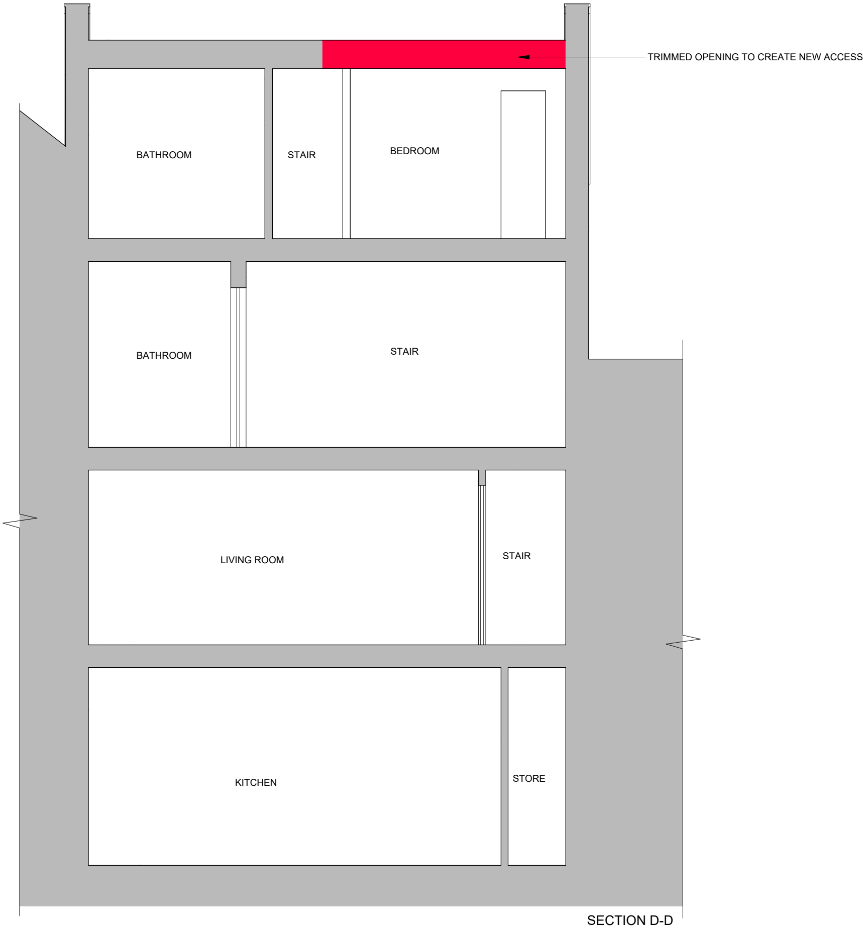
SECTION D-D
