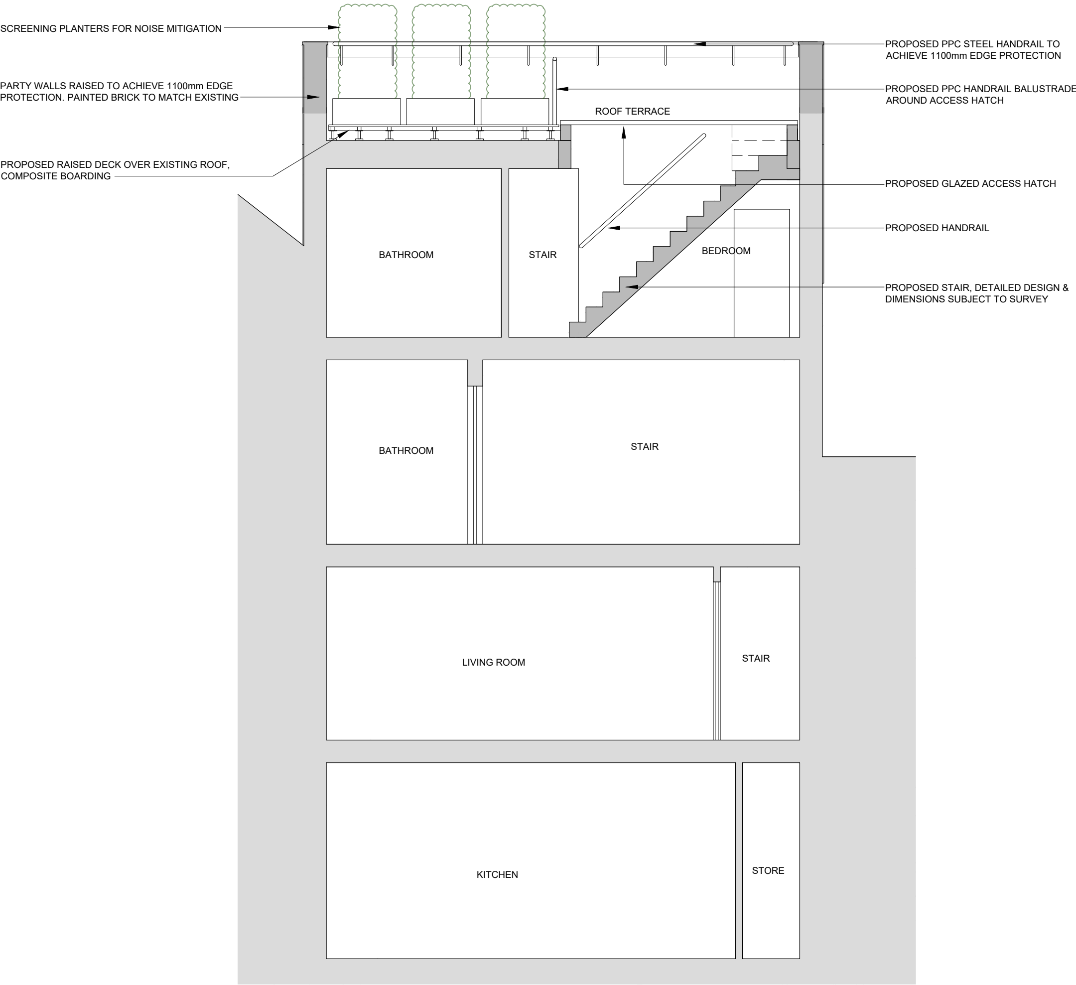
SECTION D-D
