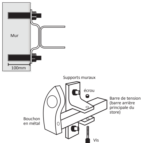
vue de côté de l'ajustement 1
