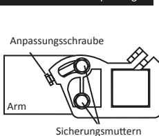
Seitenansicht auf Anpassung 1
