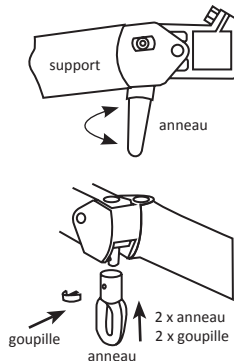
vue de côté de l'ajustement 2
