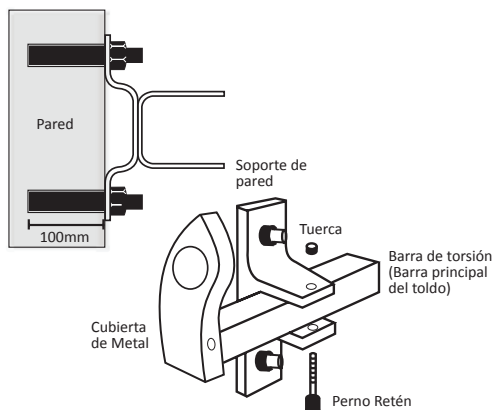
Vista lateral de ajuste 1
