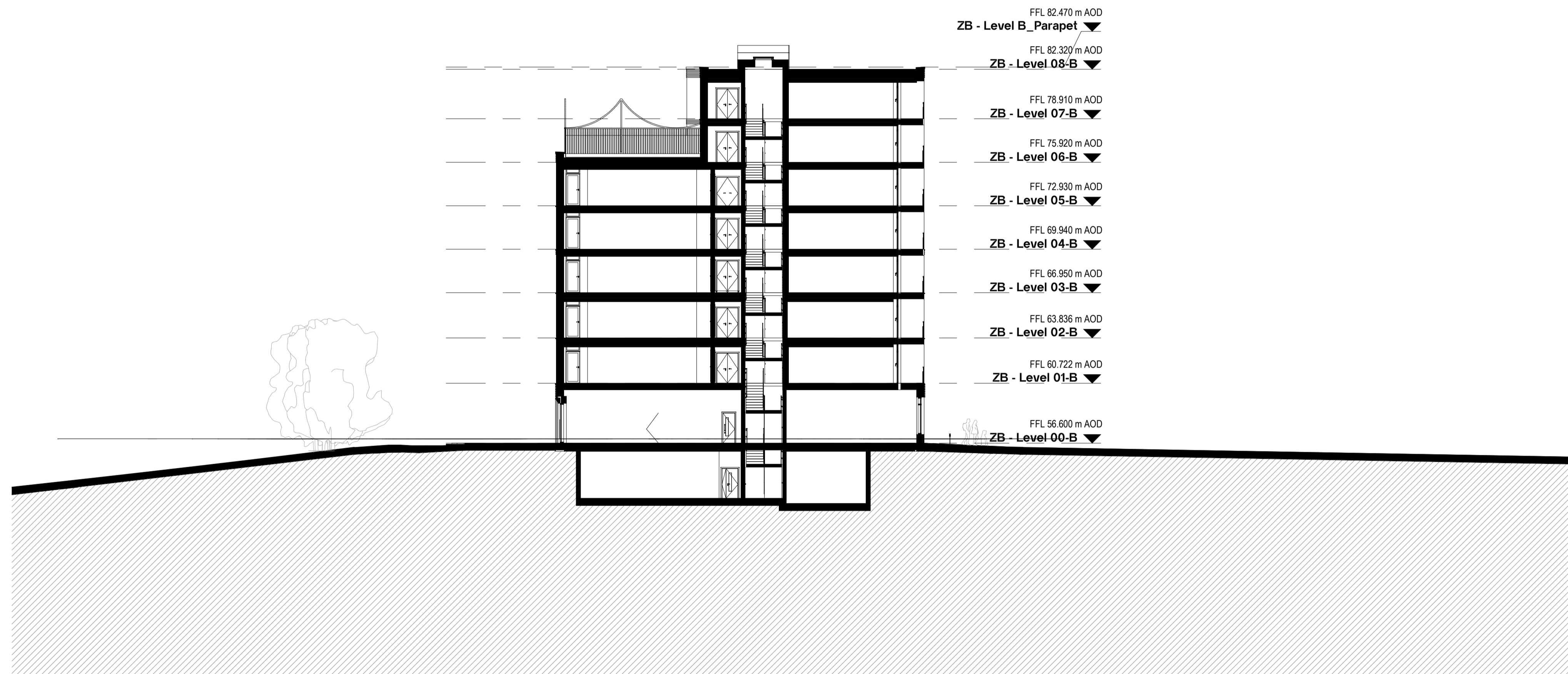
Section E-E 1 : 200
