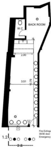
1 FLOOR PLAN 1 : 100
