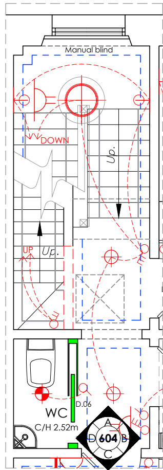
604 Floorplan 1:50
