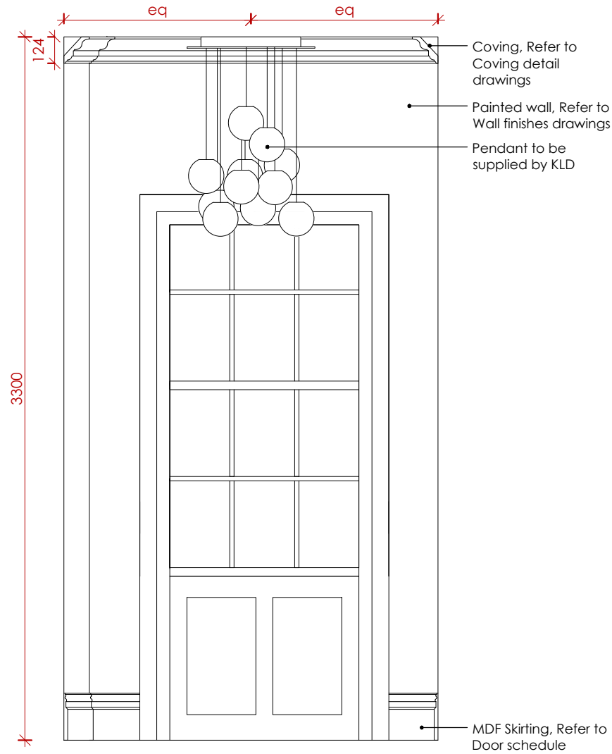
A 604 Elevation A 1:25
