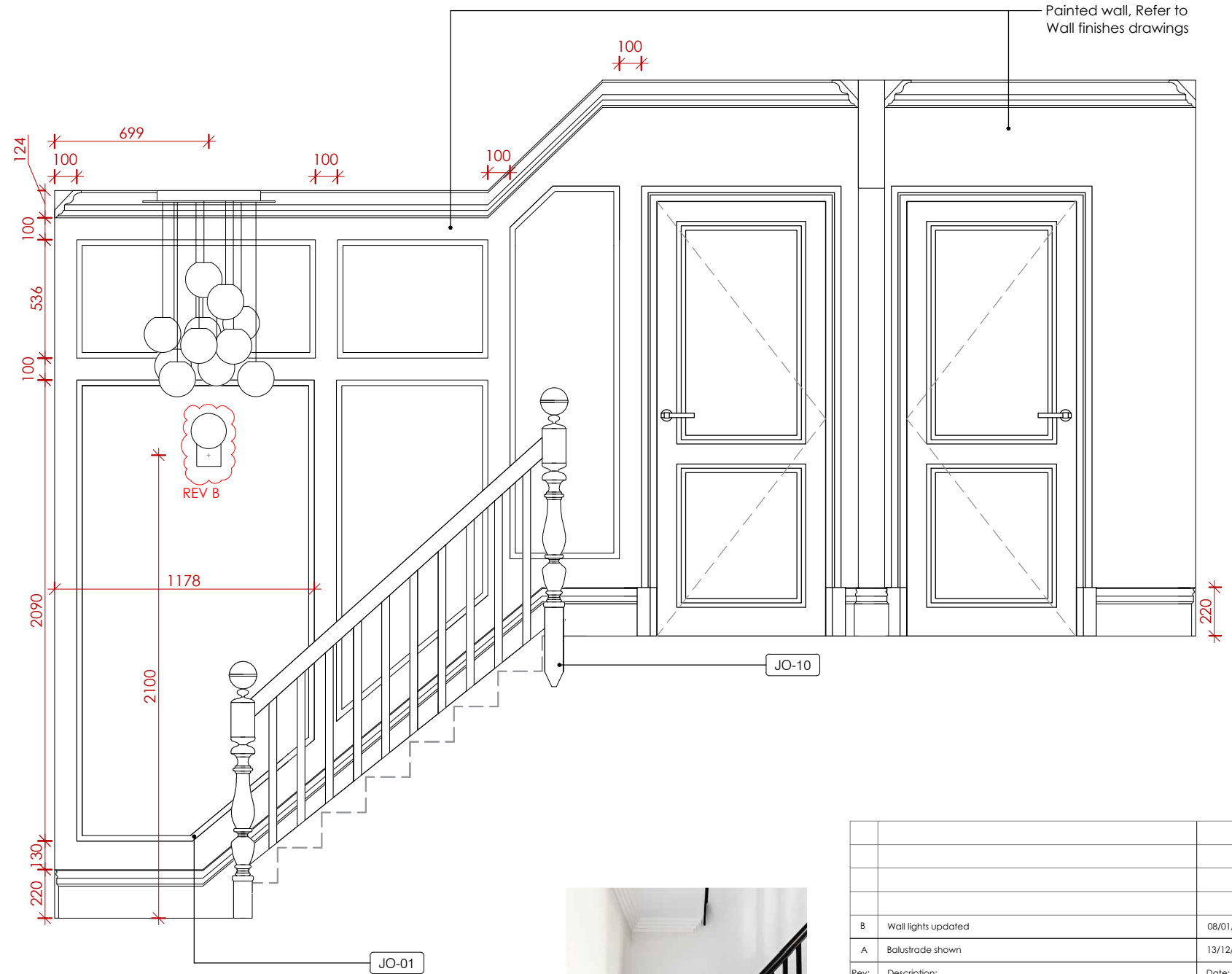
B 604 Elevation B 1:25
