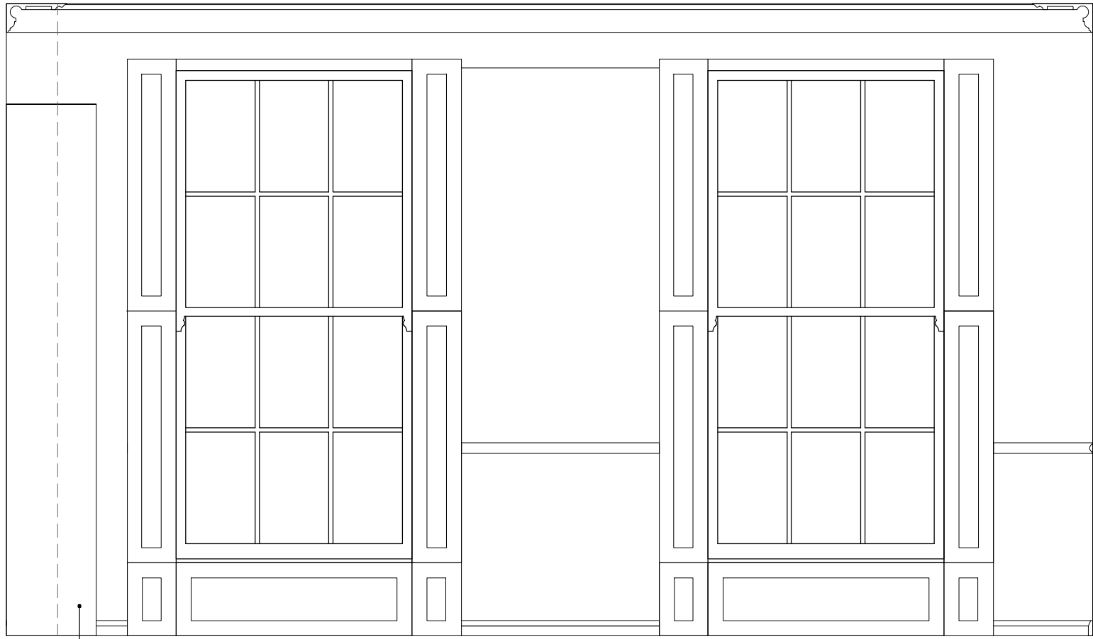
C Elevation C 652.2 1:25
