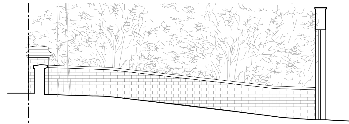
4 EXISTING ELEVATION CC 1:50 @ A3
