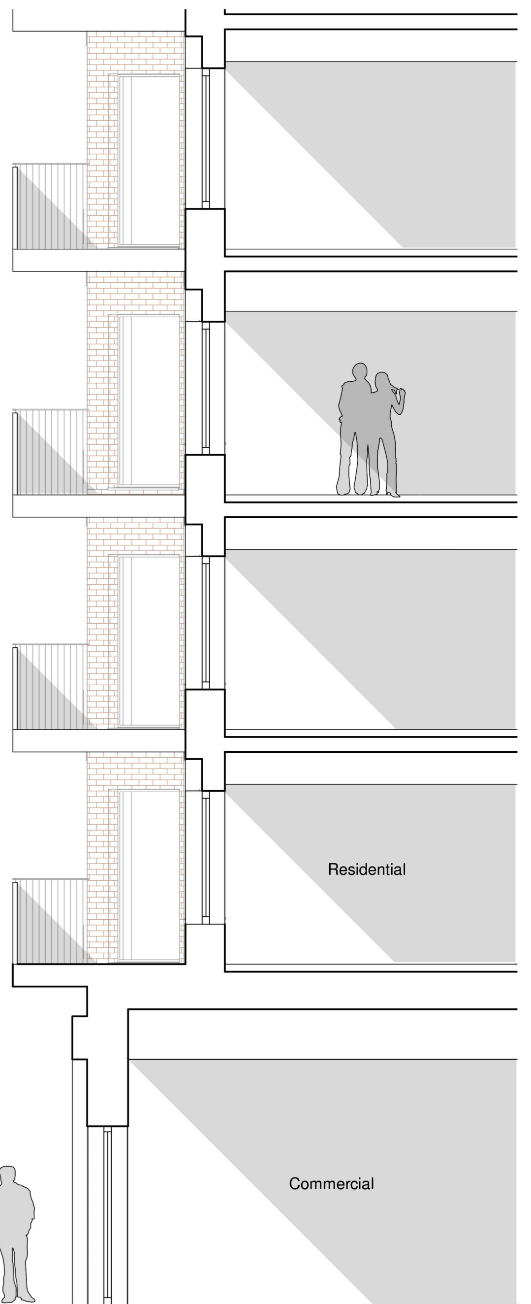
2 N3E SECTION 1 : 50
