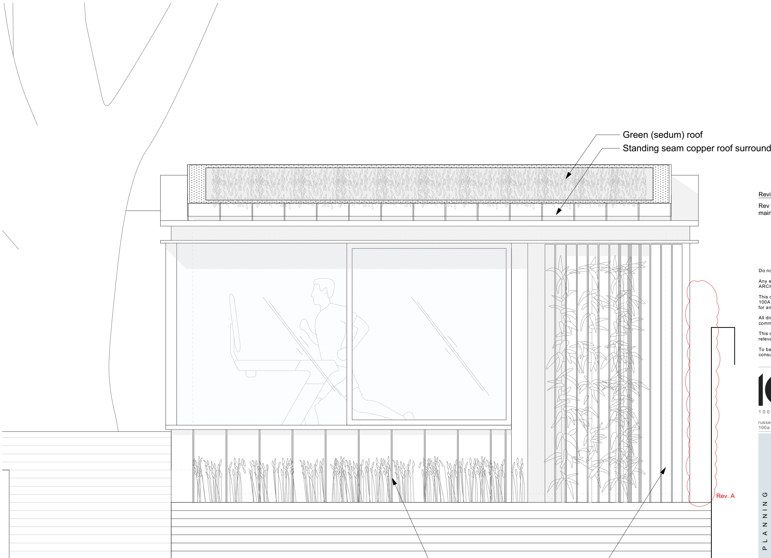
1 Front Elevation Scale: 1:20
