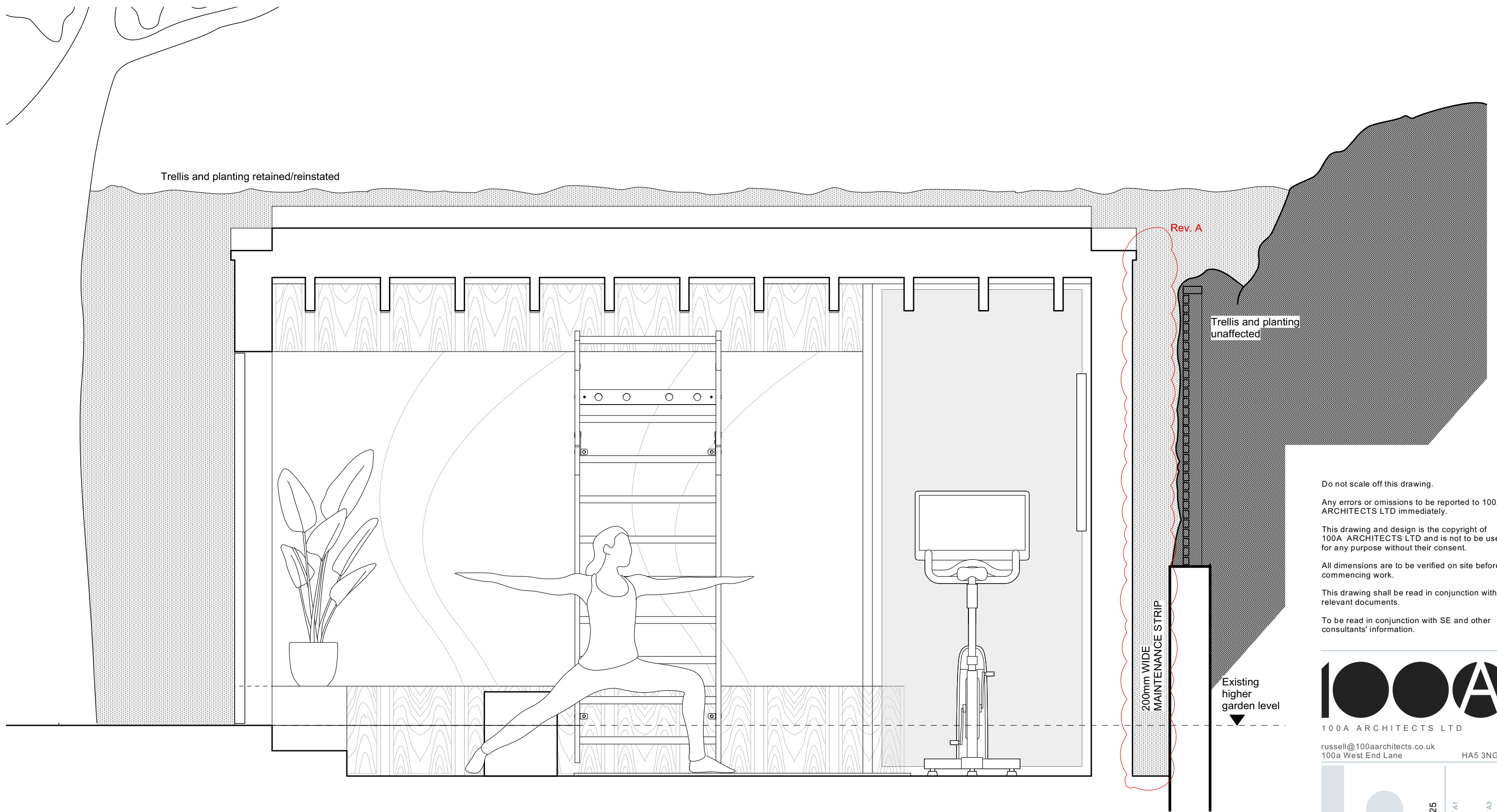
1 Section A-A Scale: 1:20
