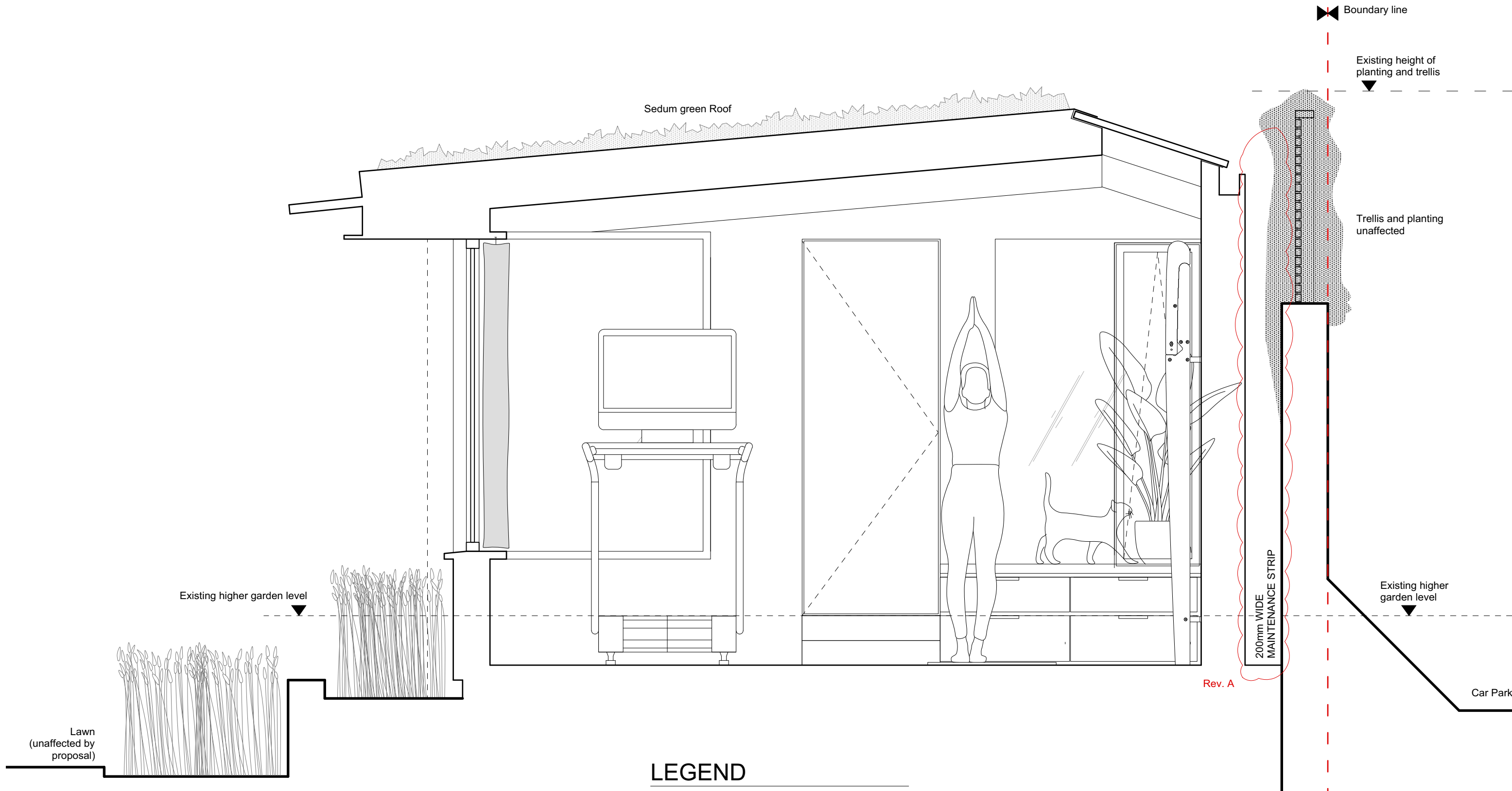
1 Section B-B Scale: 1:20
