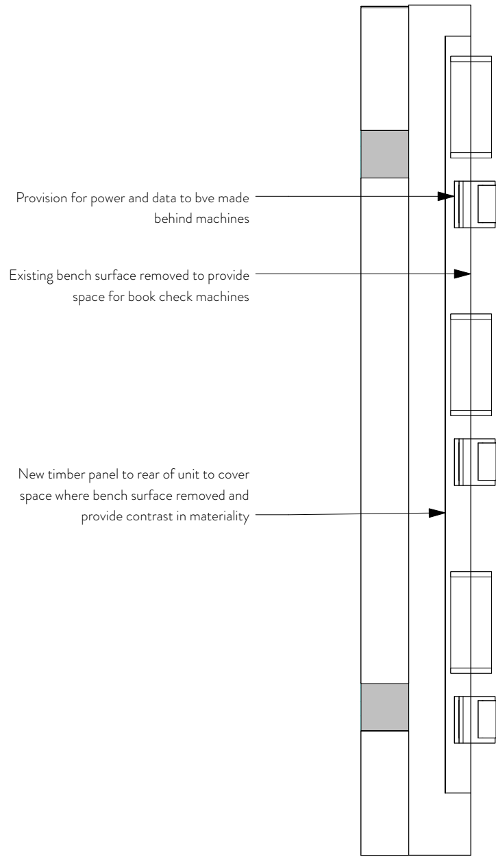
1 Level E Book Check Scale: 1:50
