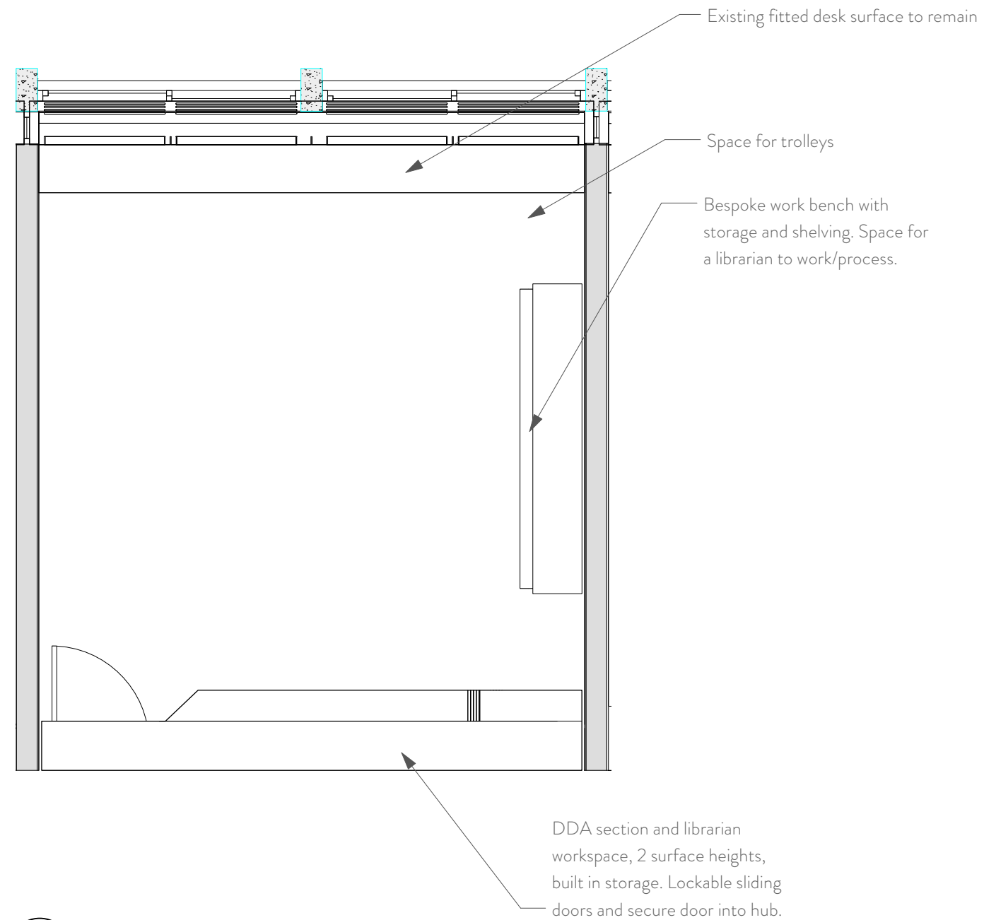
1 Level D Librarian Hub Scale: 1:50
