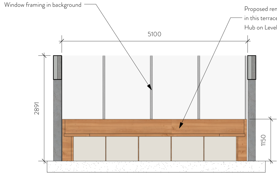
1 Front Elevation Scale: 1:50
