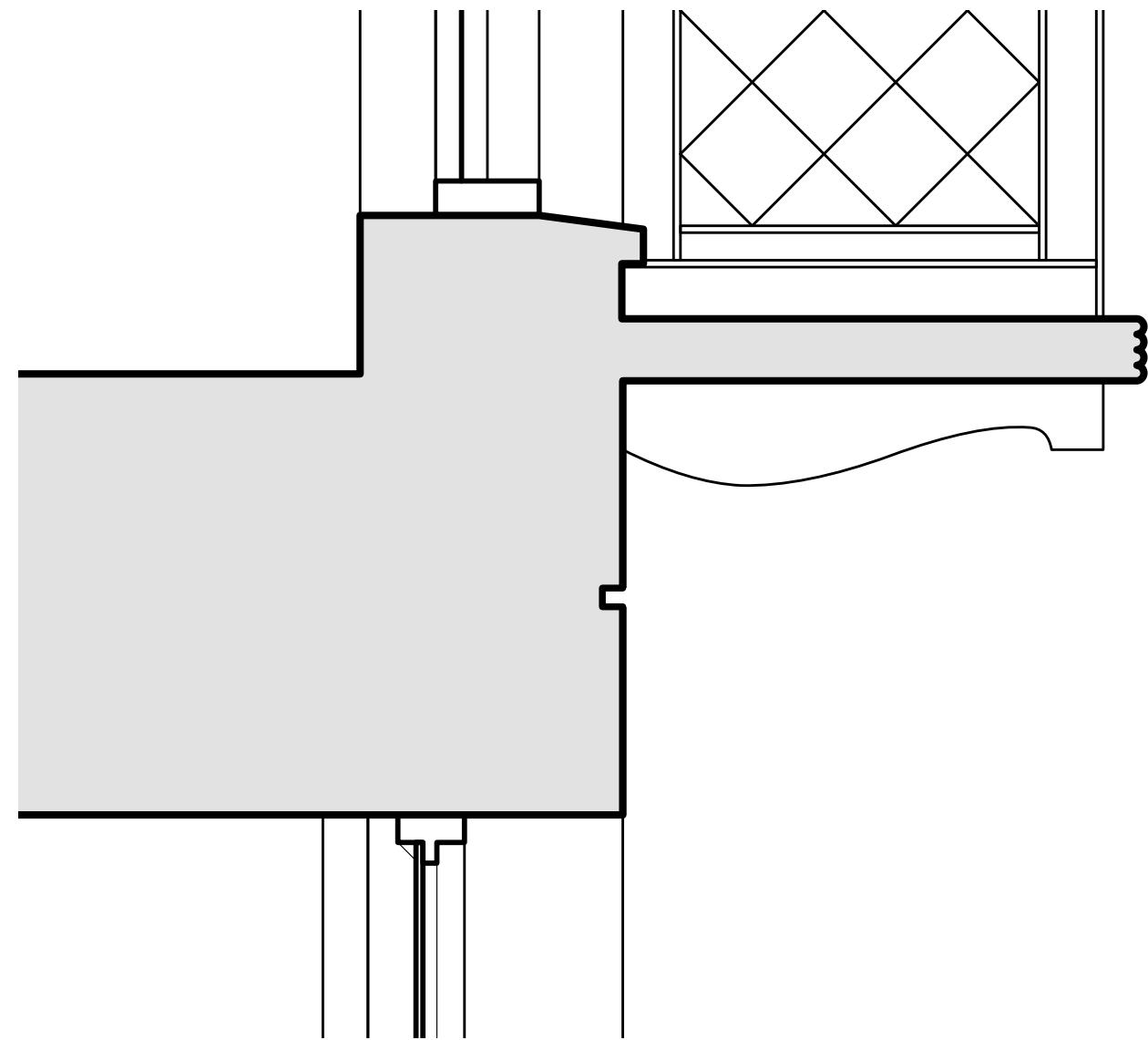
3 Existing Section AA Scale: 1:10
