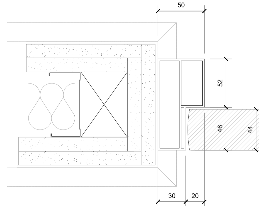
S JAMB DETAIL S 1:2
