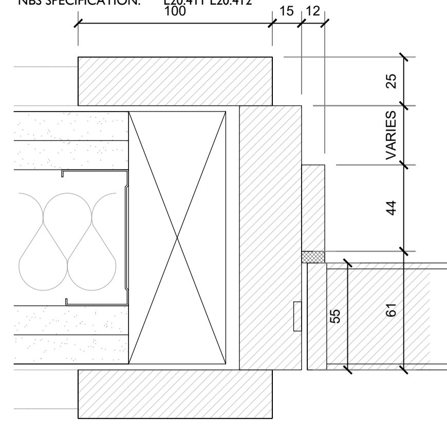
P JAMB DETAIL P 1:2
