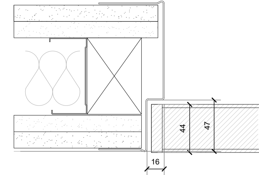
Q JAMB DETAIL Q 1:2
