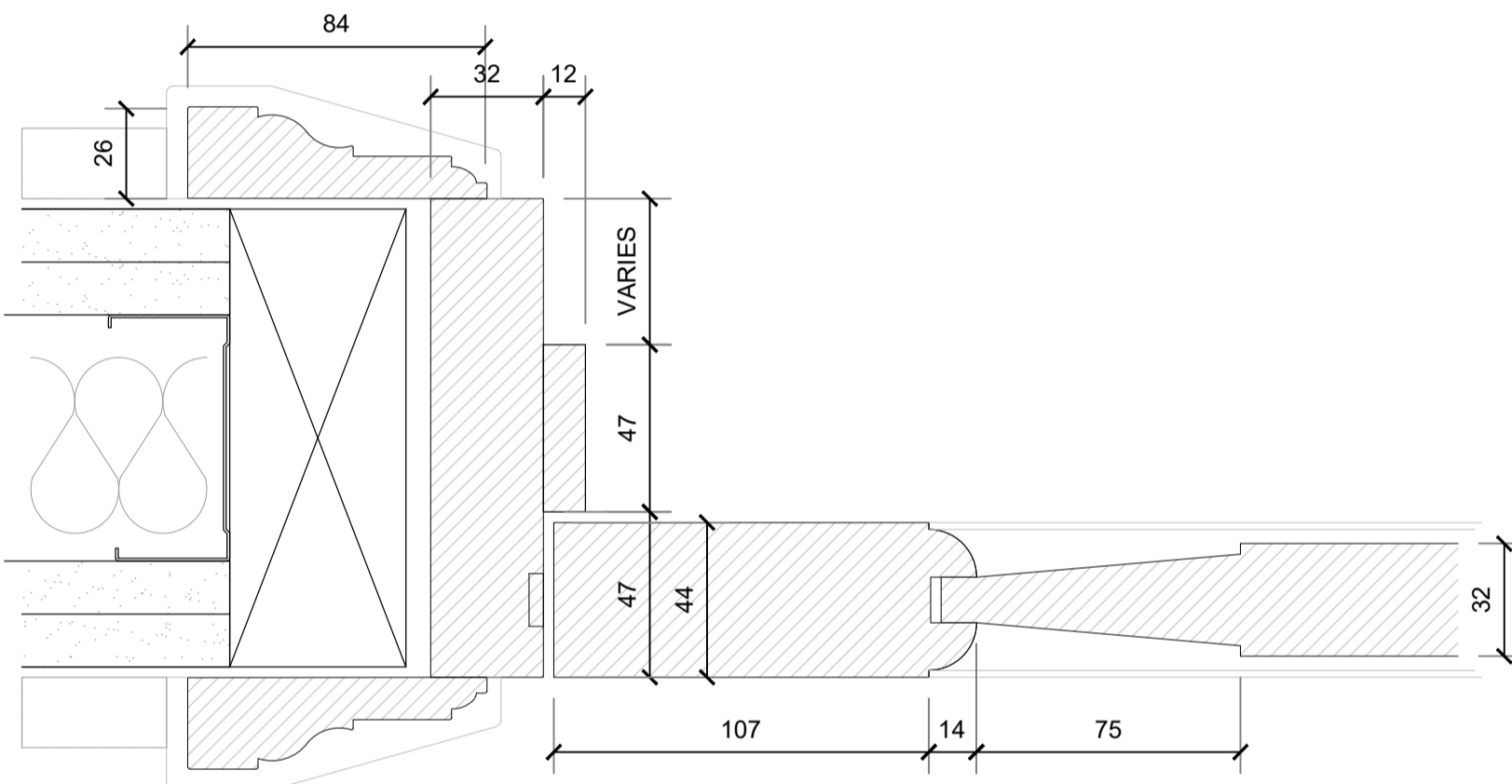
R JAMB DETAIL R 1:2
