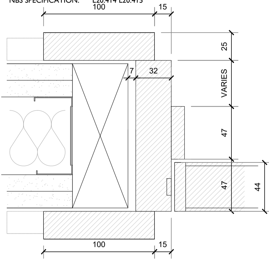
O JAMB DETAIL O 1:2
